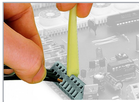
Geleider aansluiten - met bedieningsgereedschap.
