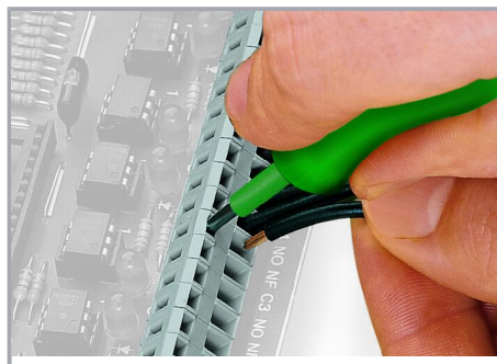
Geleider aansluiten - met schroevendraaier (bladbreedte 3,5 mm).
