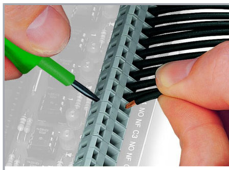
Geleider aansluiten - met schroevendraaier (bladbreedte 3,5 mm).
